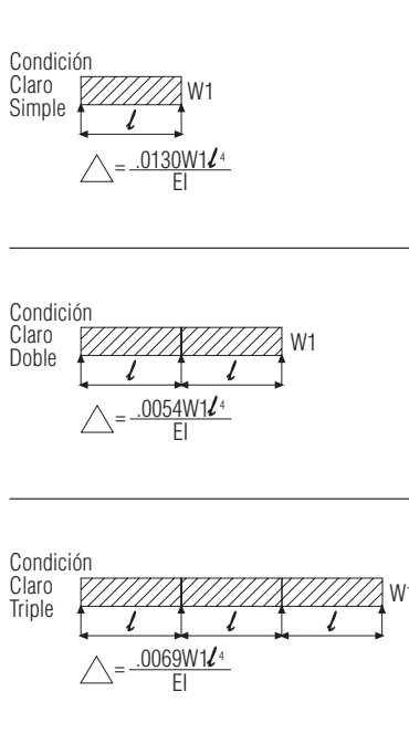
FIG. 2 Diagramas de cargas para deflexiones
