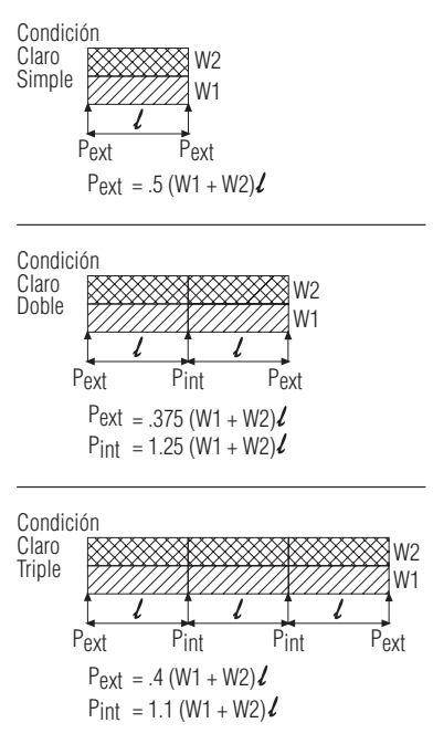
FIG. 3 Diagramas de cargas para reacciones en los apoyos
